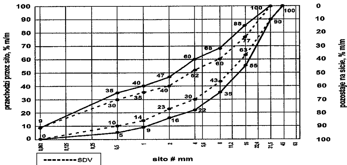
Rys. 1. Krzywe graniczne uziarnienia mieszanki niezwiązanej z kruszywem C50/30 do warstw podbudowy
