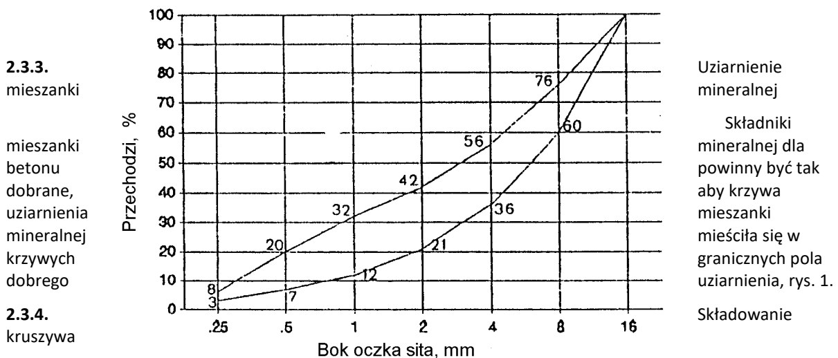
Rysunek 1. Krzywe graniczne uziarnienia kruszywa do betonu
