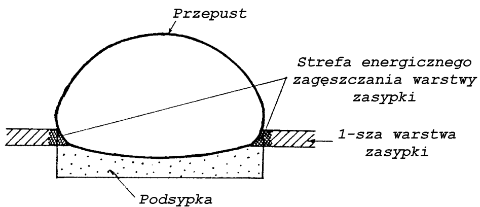
Przykład wykonania pierwszej warstwy zasyпки po zmontowaniu przepustu z blachy falistej
