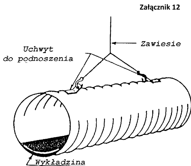
Przykład transportu odcinka zmontowanego przepustu z blach falistych za pomocą dźwigu
