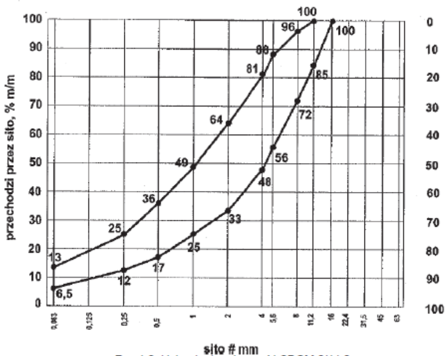
Rys.1.2. Uziarnienie mieszanki CBGM 0/11,2
