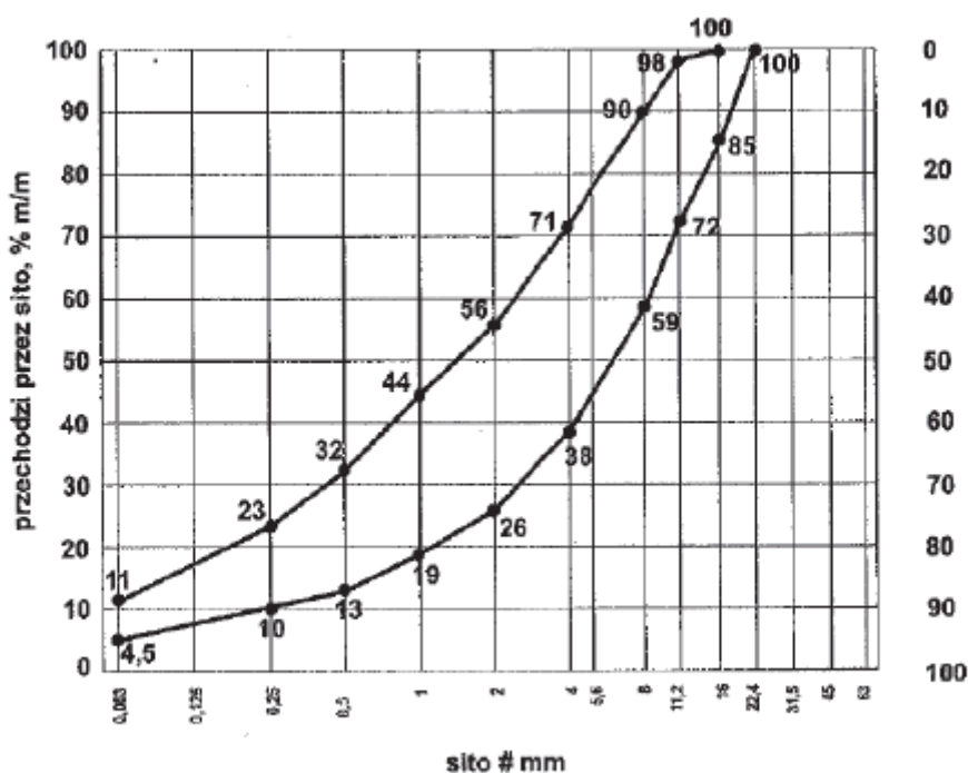
Rys.1.2. Uziarnienie mieszanki CBGM 0/16
