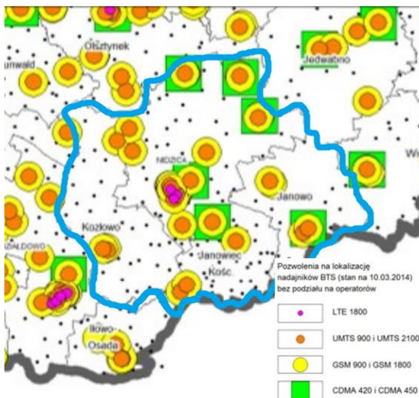
Rycina 13. Przekazniki stacje bazowe (BTS)
